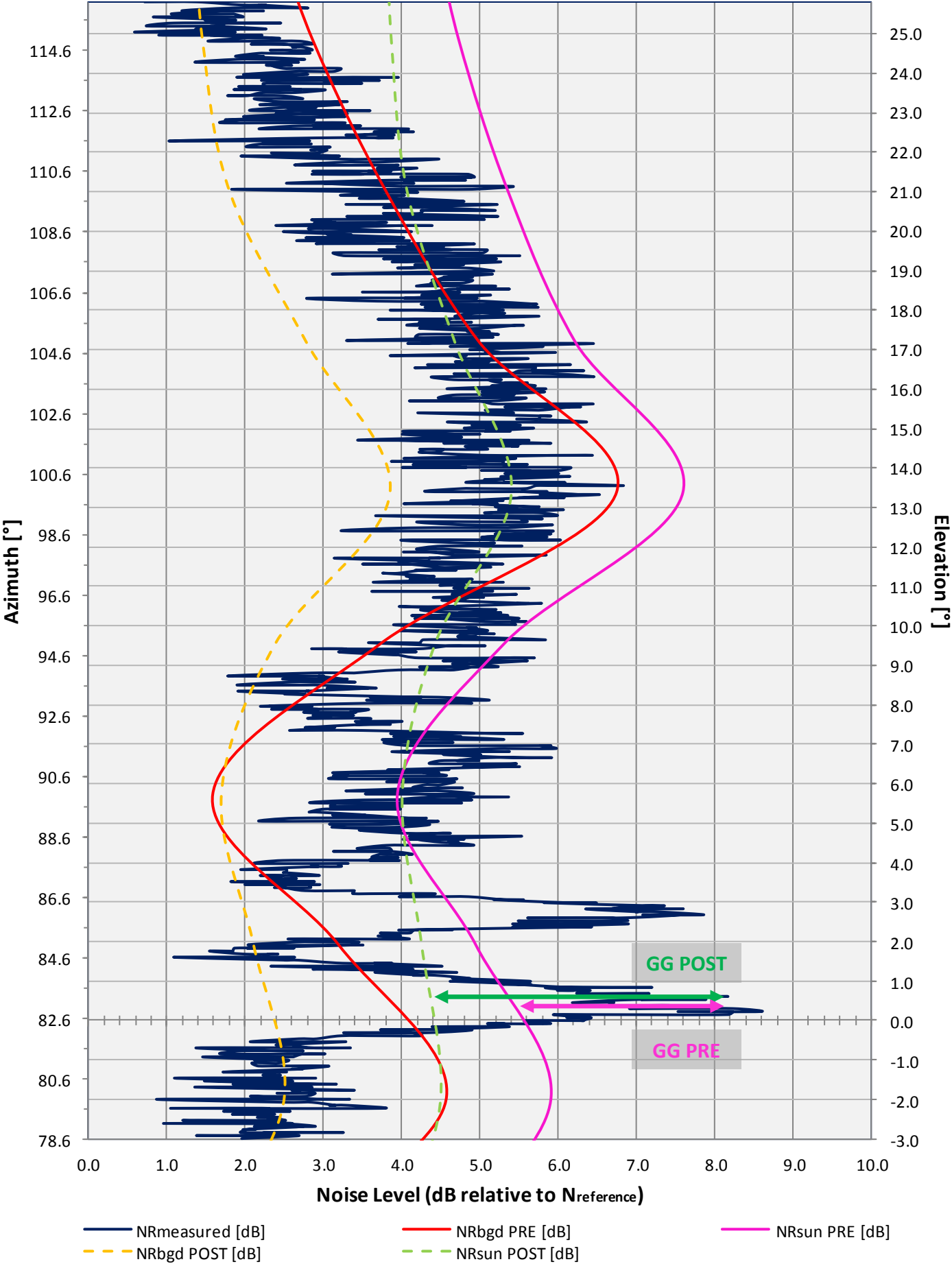
Fig. 27 : Sun rise measurement
